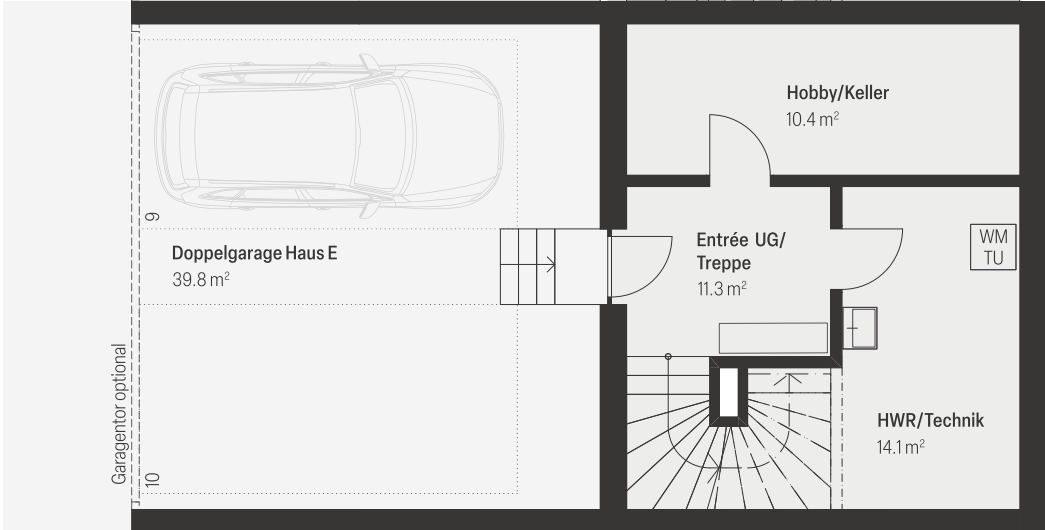
Untergeschoss
