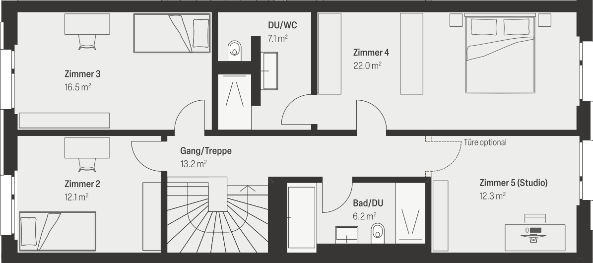
Obergeschoss
